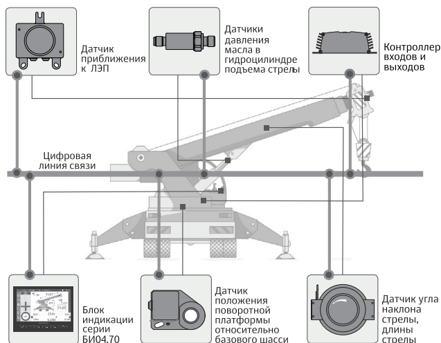
Рисунок 1. Структурная схема ОГМ240
