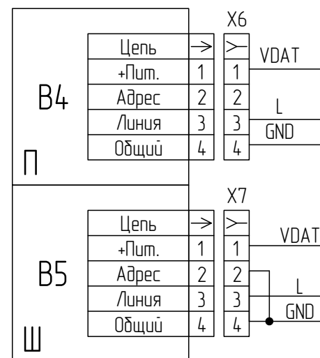
Датчики избыточного давления в гидроцилиндре подъема стрелы
