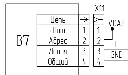
Датчик избыточного давления в гидросистеме крана
