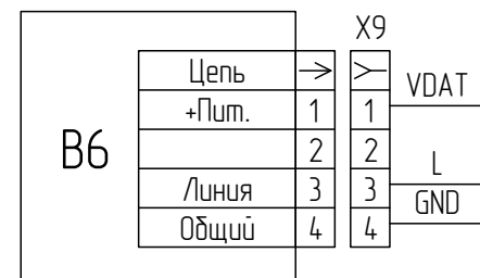
Датчик азимута
